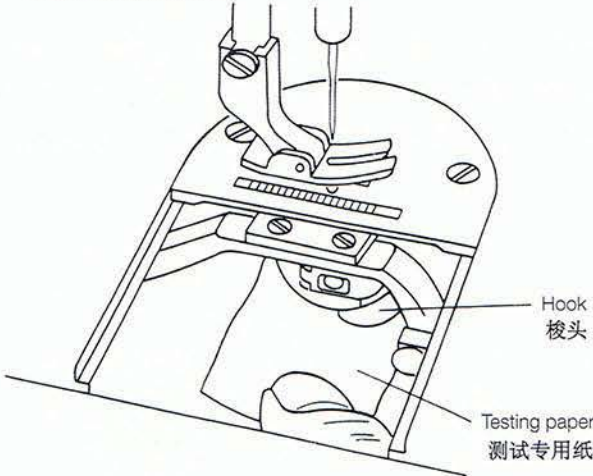
Fig.1 : How to check state of lubrication 查看润滑状况的方法
